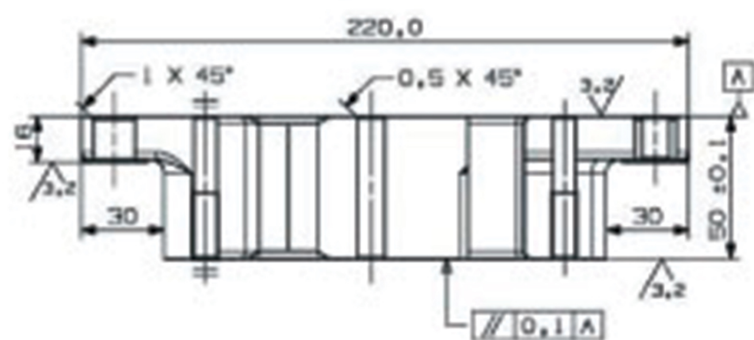
SECTION A-A
